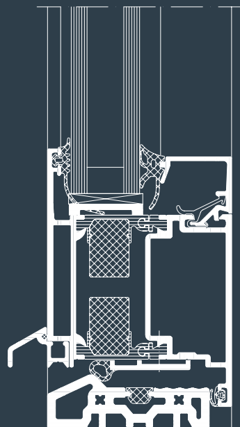
Schüco Tür ADS 70.HI, Fußpunkt, Maßstab 1:2 Schüco Door ADS 70.HI, sill, scale 1:2
