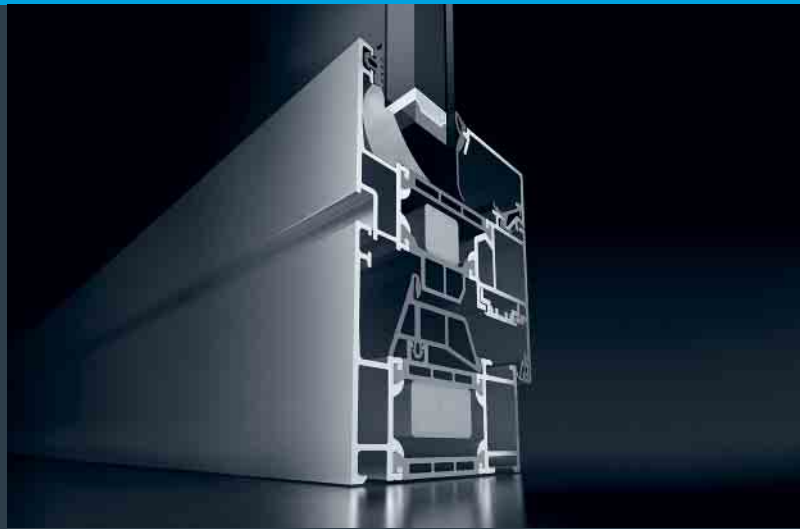
Schüco Fenster AWS 70.HI mit WK2 Schüco Window AWS 70.HI with WK2
